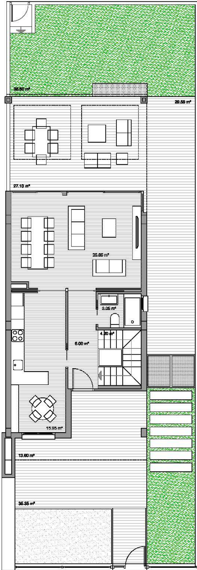
PLANTA BAJA
