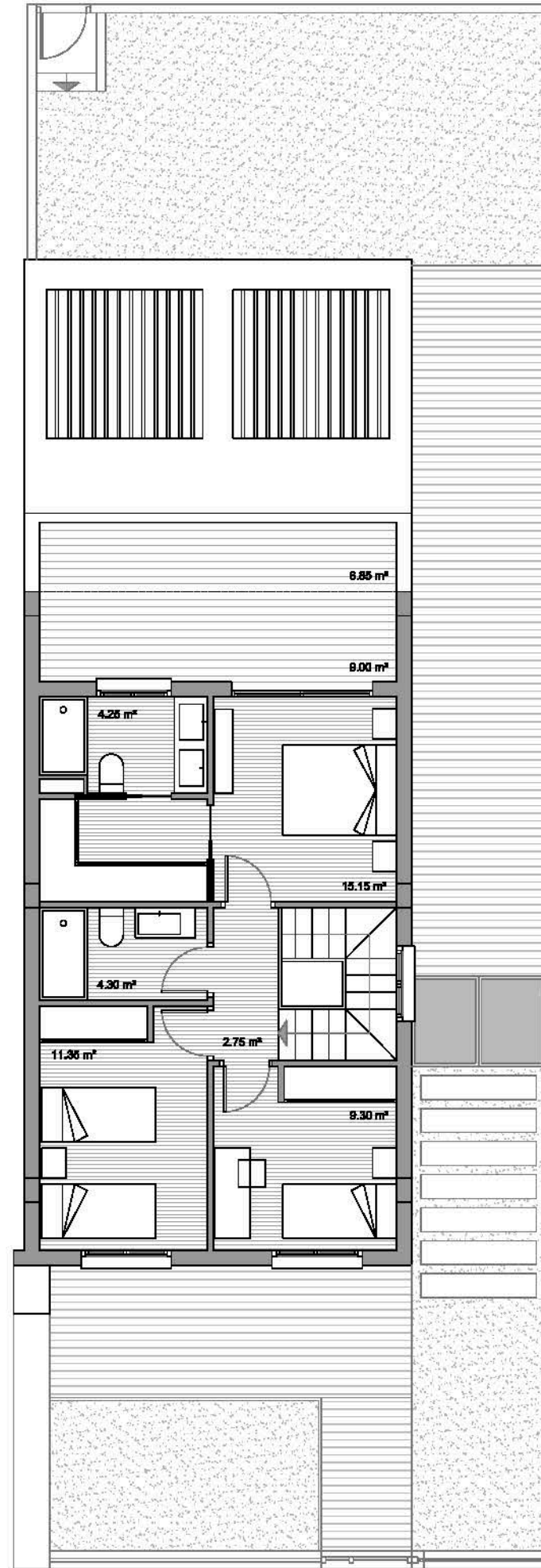
PLANTA PRIMERA
